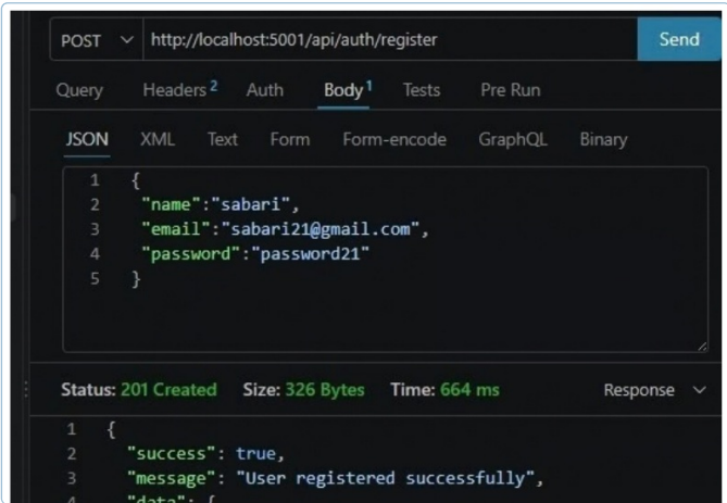
Register - 201 Created, 326 Bytes, 664 ms
