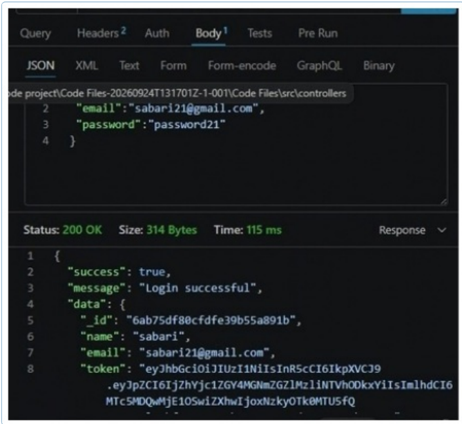
Login - 200 OK, 314 Bytes, 115 ms
